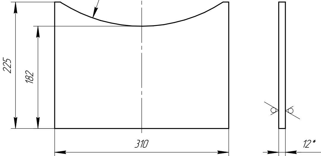
Дет. поз. 3
