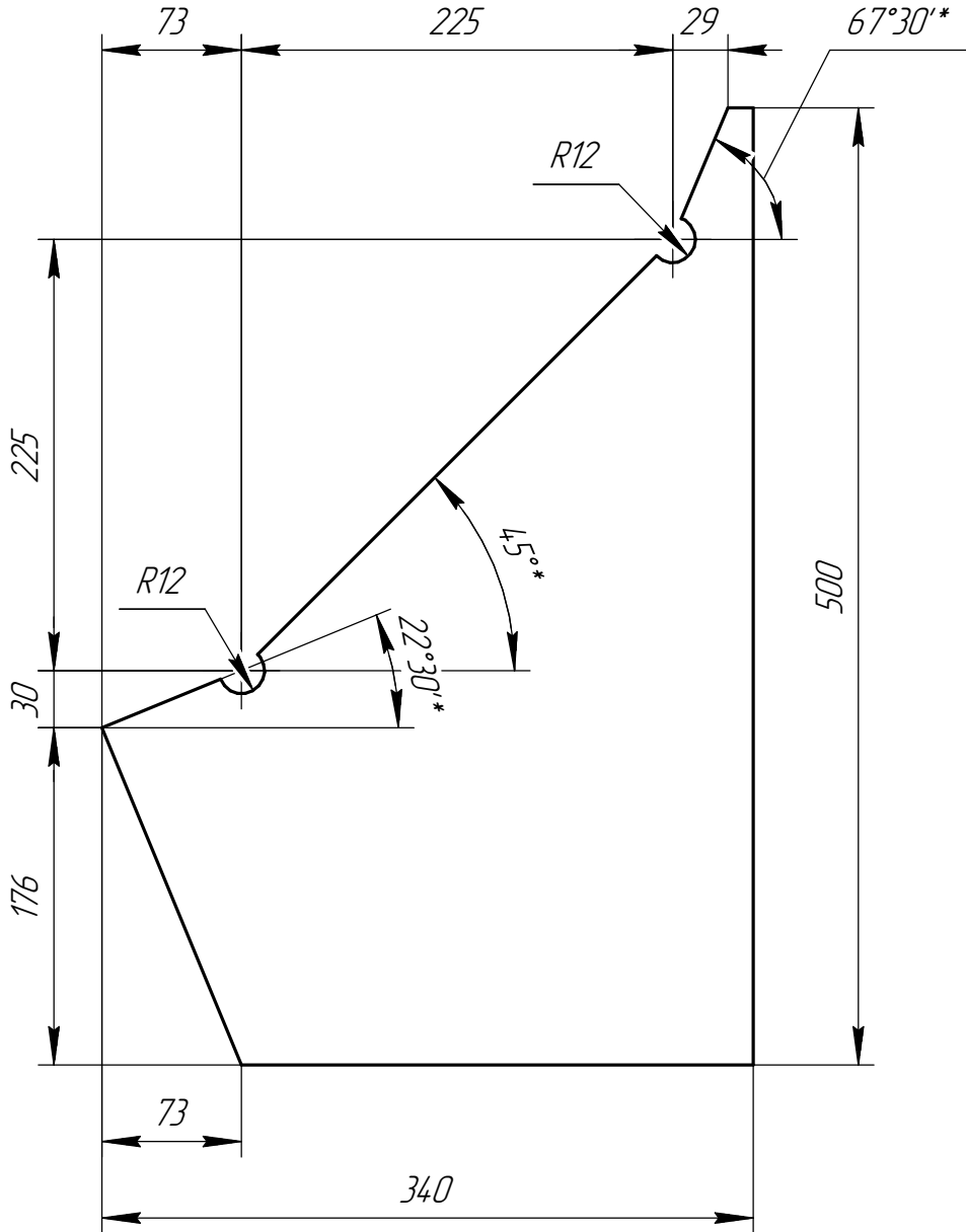
Дет. поз. 1
